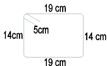
Εικόνα 7: Συνδετήρας για εγκάρσιο οπλισμό διαζώματος που τοποθετείται ανά 10 εκατοστά.
