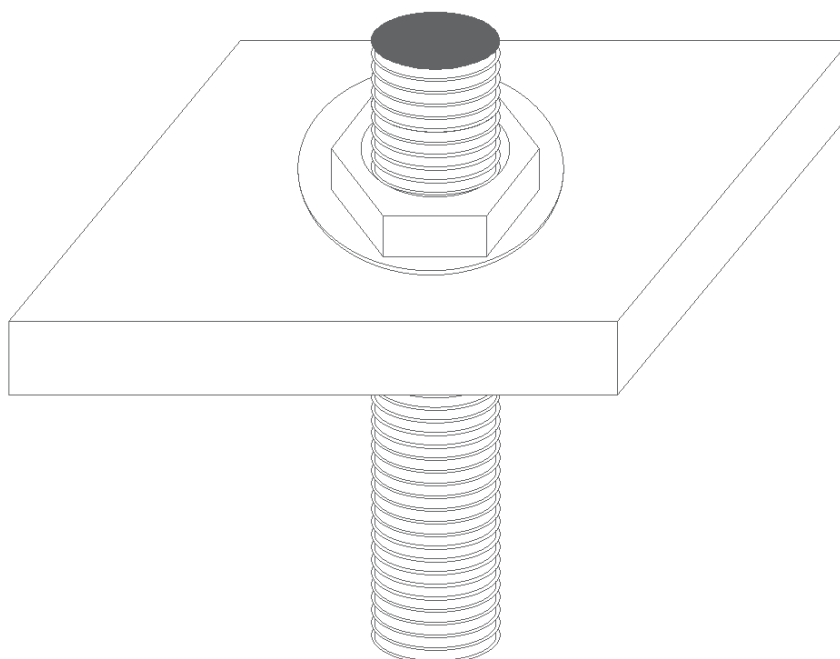
Εικόνα 5: Διάταξη αγκυρίου - πλάκας αγκύρωσης - ροδέλας - περικοχλίου.
