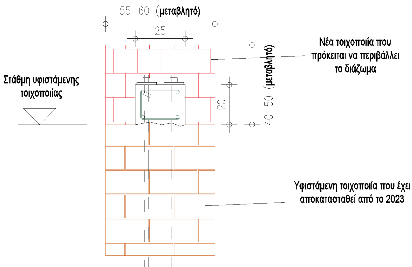
Εικόνα 10: Κατασκευή τοιχοποιίας πάνω από την στέψη του υφιστάμενου τείχους για την ενσωμάτωση του διαζώματος οπλισμένου σκυροδέματος.
