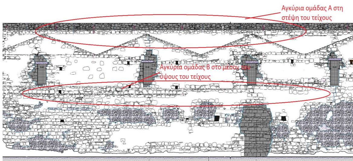
Εικόνα 3: Όψη τείχους από αρχιτεκτονικά σχέδια αποκατάστασης, στην οποία διακρίνονται οι δύο βασικές ομάδες αγκυρίων.
