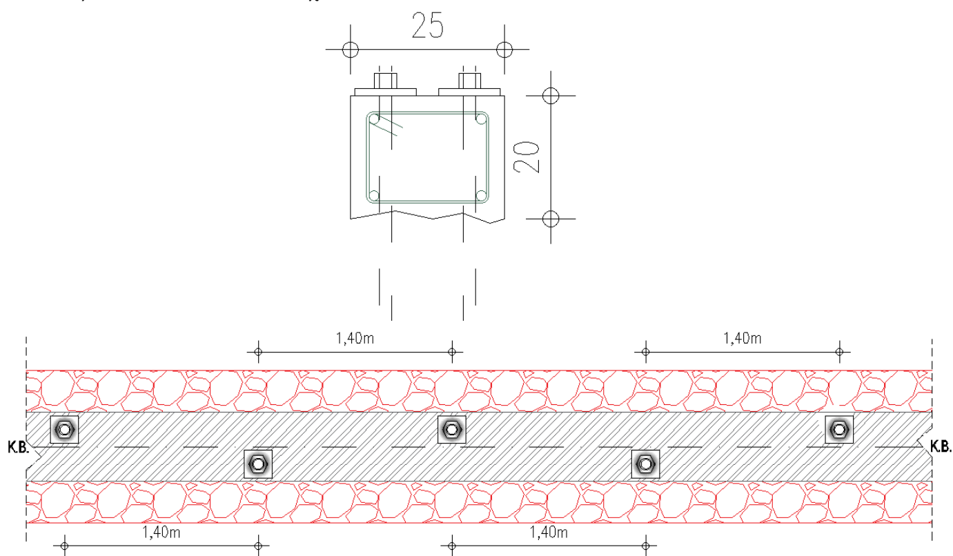
Εικόνα 4: Κατακόρυφα αγκύρια ομάδας Α τοποθετημένα στην στέψη του τείχους, ανά 1,40 m σε εναλλάξ διάταξη (όπως φαίνεται στην κάτοψη) με μήκος 4,30 m έκαστο.
