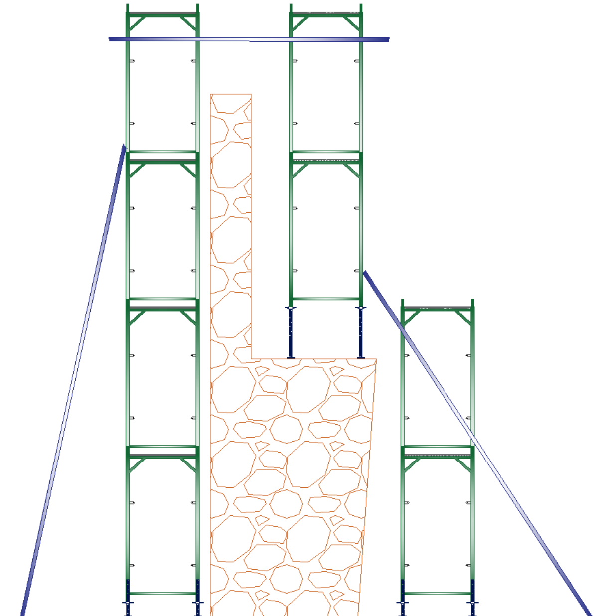
Εικόνα 9: Σκαρίφημα 2, με ενδεικτικό τρόπο τοποθέτησης ικριωμάτων στο ανατολικό τμήμα του τείχους που έχει μεγαλύτερο πάχος στη βάση (μεταβλητό, περίπου 2,20 m ) και αρνητική κλίση.
