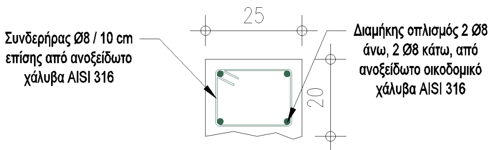
Εικόνα 6: Διάζωμα από οπλισμένο σκυρόδεμα στην στέψη του τείχους, σε τομή.
