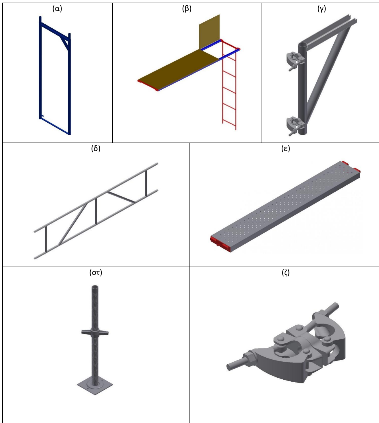
Πίνακας 6: Βασικά τμήματα ικριωμάτων για την εξασφάλιση της ασφαλούς λειτουργίας ((α)πλαίσιο ύψους 2 μέτρων, (β) πλατφόρμα εργασίας με σκάλα, (γ) πρόβολος για προέκταση της σκαλωσιάς σε σημεία που δεν δύναται να τοποθετηθούν πλαίσια, (δ) προστατευτική πλάτη, (ε) δάπεδο από αντιολισθητική λαμαρίνα πλάτους 30 εκατοστών, τοποθετούνται 3 ανάμεσα σε δύο αντικριστά πλαίσια, (στ) βίδα «κάτω» με χαρακτηριστικό της την πλάκα στη βάση της και χρησιμοποιείται για την έδραση των πλαισίων, (ζ) σύνδεσμος είτε σταθερής είτε μεταβλητής γωνίας)
