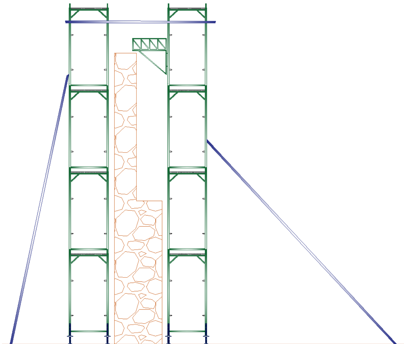
Εικόνα 8: Σκαρίφημα 1, με ενδεικτικό τρόπο τοποθέτησης ικριωμάτων στο δυτικό τμήμα του τείχους που έχει μικρότερο πάχος στη βάση (περίπου 1,20 m).
